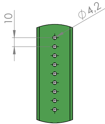
DÉTAIL Q ECHELLE 2 : 5
